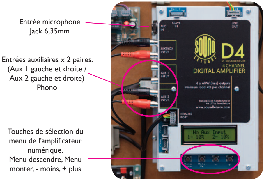
FIG 8 VUE DE L'AMPLIFICATEUR NUMÉRIQUE D4
