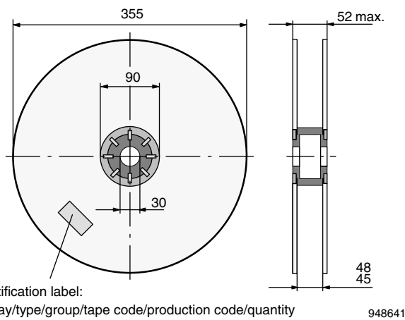
Fig. 18 - Reel
